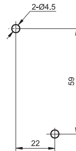
安装孔尺寸图
